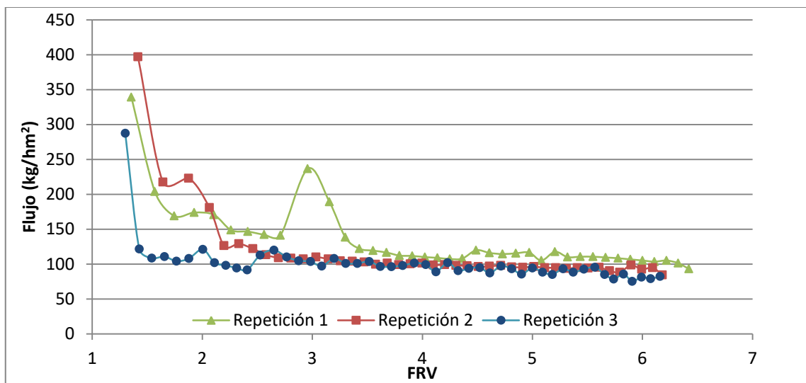
Figura 37. Flujo de permeado respecto al FRV en la ultrafiltración de licor de pescado en una membrana de 50 nm (Temperatura: 60 °C; P_{tm} : 1,2-1,4 bar).
