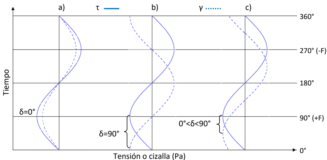
Figura 6. Relación de \tau y \gamma respecto al tiempo y \delta de acuerdo al comportamiento del material: a) elástico ideal, b) viscoso ideal y c) viscoelástico.
