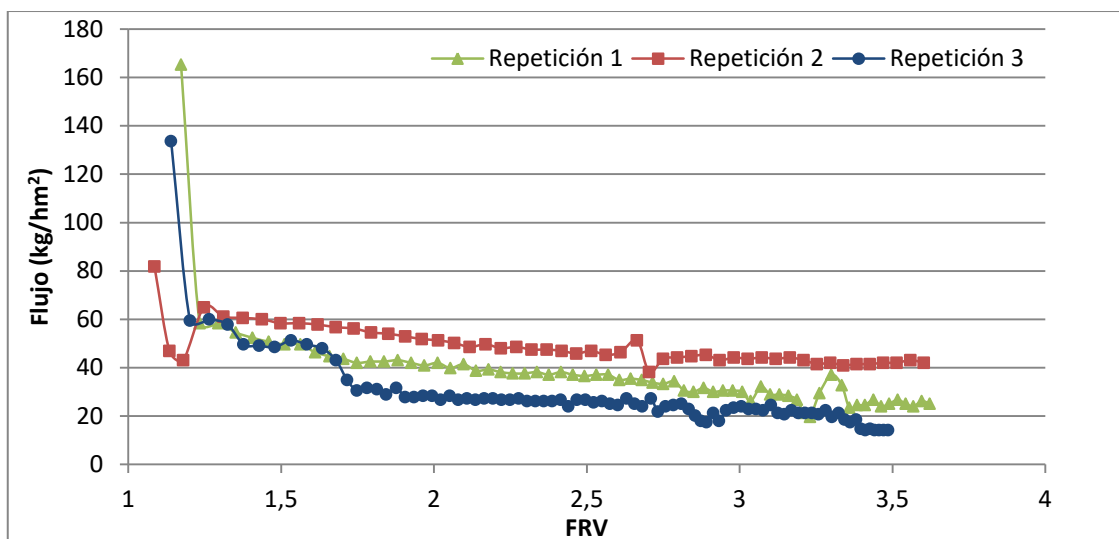
Figura 39. Flujo de permeado respecto al FRV en la ultrafiltración de licor de pescado en una membrana de 20 nm (Temperatura: 60 °C; P_{tm} : 1,6-1,8 bar).
