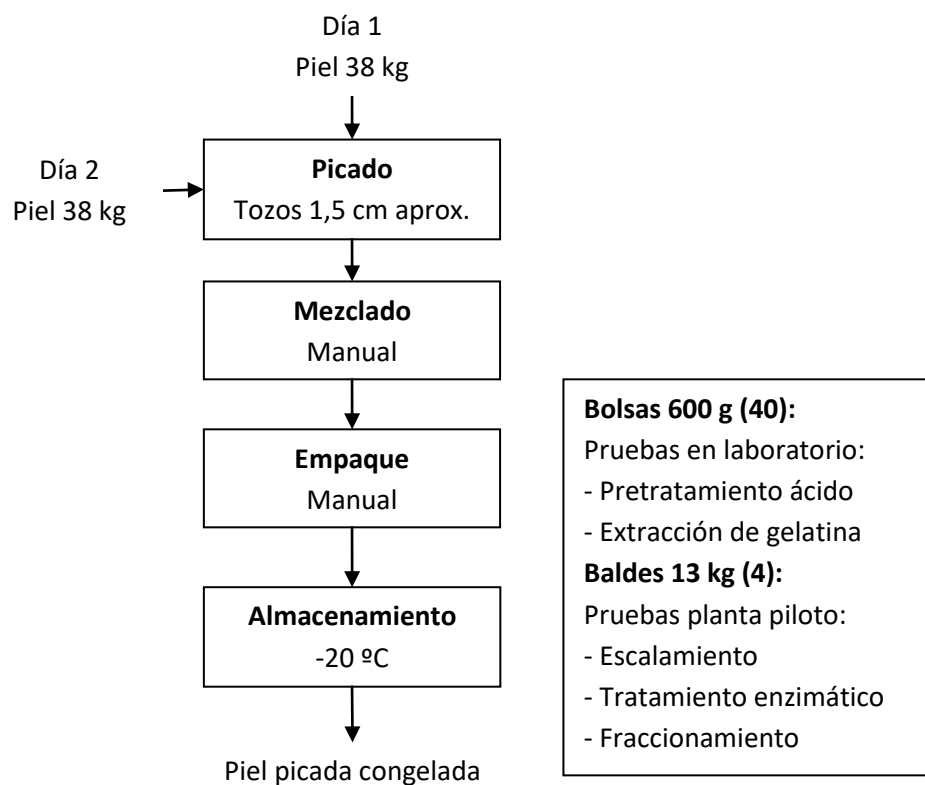
Figura 15. Flujo de proceso para la preparación de la piel de atún para realizar las pruebas a nivel de laboratorio y de planta piloto.
