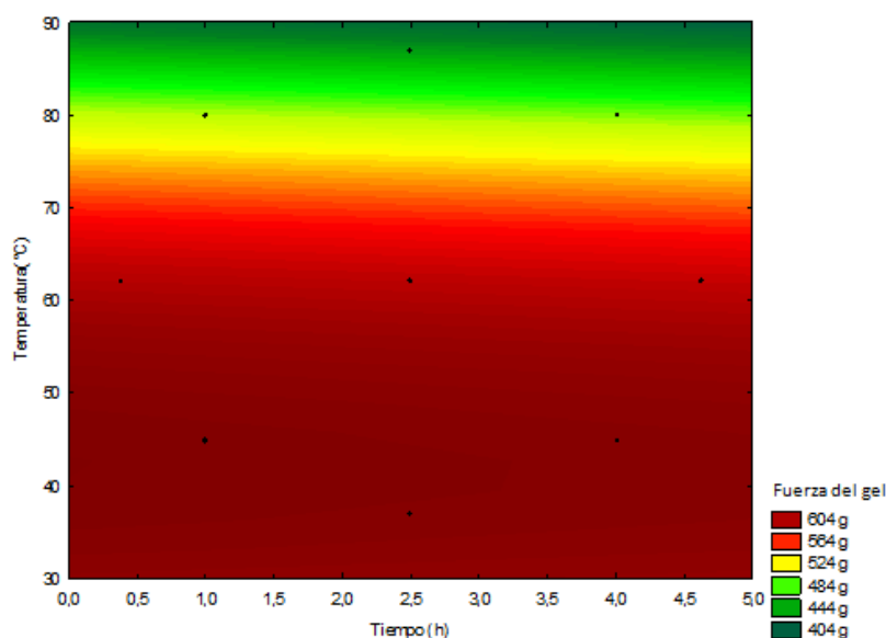
Figura 27. Efecto del tiempo y de la temperatura de extracción sobre la fuerza del gel elaborado con la gelatina extraída de la piel de atún.
