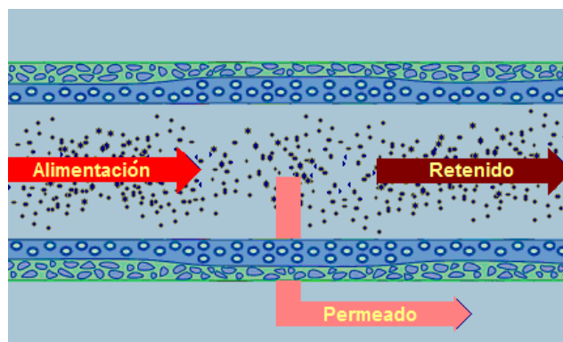
Figura 12. Principio de filtración tangencial. Fuente GEA (2007).
