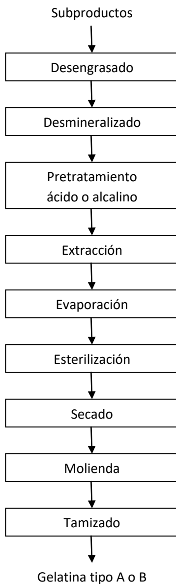
Figura 4. Proceso convencional para la obtención de gelatina. Adaptado de Karayannakidis y Zotos (2016).
