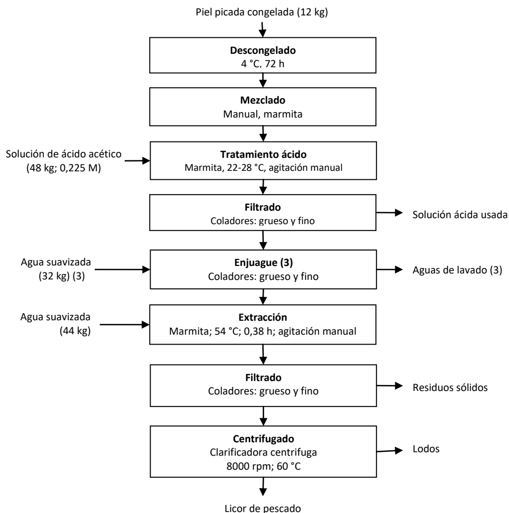
Figura 17. Flujo de proceso de la extracción del licor de pescado a escala de planta piloto.
