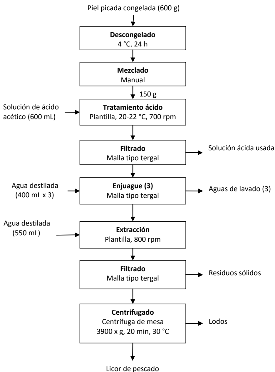
Figura 16. Flujo de proceso de la extracción del licor de pescado en el laboratorio.
