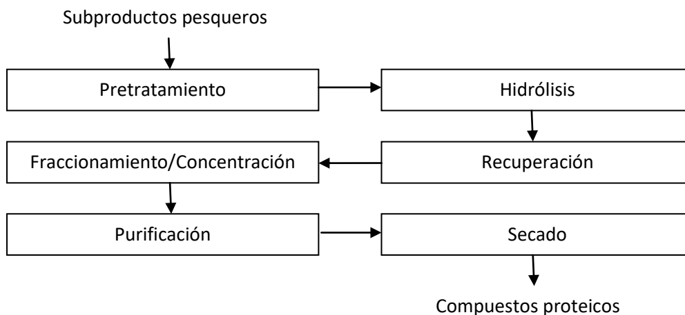
Figura 13. Proceso general para la obtención de compuestos proteicos funcionales a partir de subproductos de la industria pesquera.
