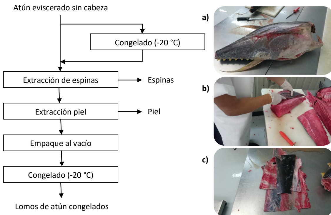
Figura 14. Flujo de proceso de elaboración de lomos de atún fresco en la empresa Tunatun S.A. Fotografías: a) atún descongelado; b) extracción de los lomos, y c) pieles de atún.
