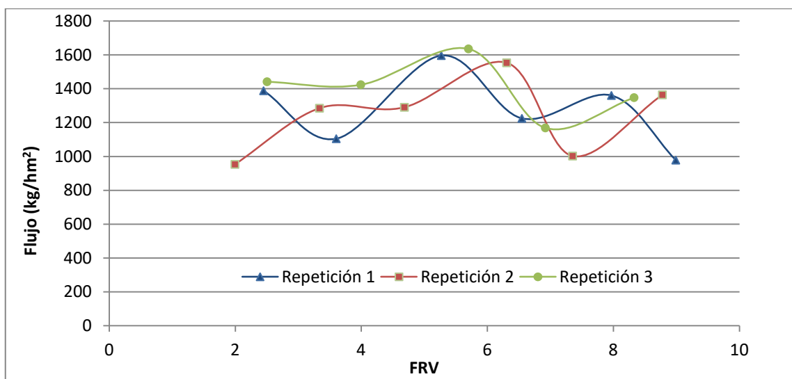
Figura 33. Flujo de permeado respecto al FRV en la microfiltración de licor de pescado en una membrana de 0,8 µm (Temperatura: 60 °C; P_{tm} : 0,7-1,0 bar).
