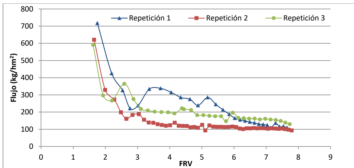
Figura 35. Flujo de permeado respecto al FRV en la ultrafiltración de licor de pescado en una membrana de 100 nm (Temperatura: 60 °C; P_{tm} : 1,2-1,4 bar).
