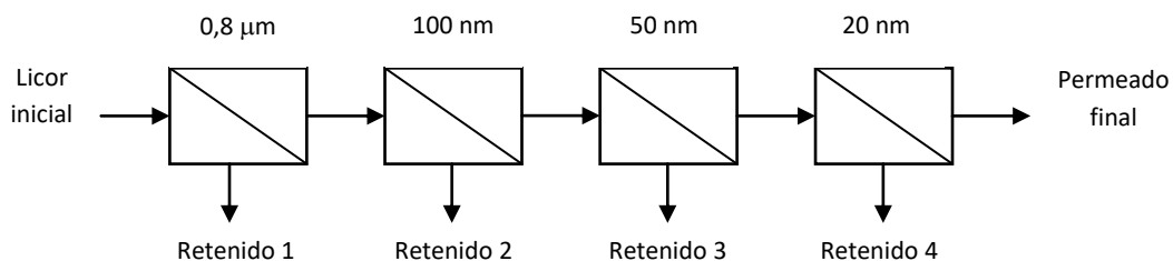
Figura 18. Diagrama del fraccionamiento de proteínas por tecnología de membranas.
