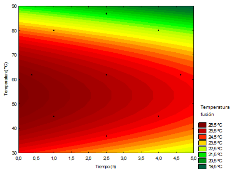
Figura 26. Efecto del tiempo y de la temperatura de extracción sobre la temperatura de fusión de la gelatina de piel de atún.
