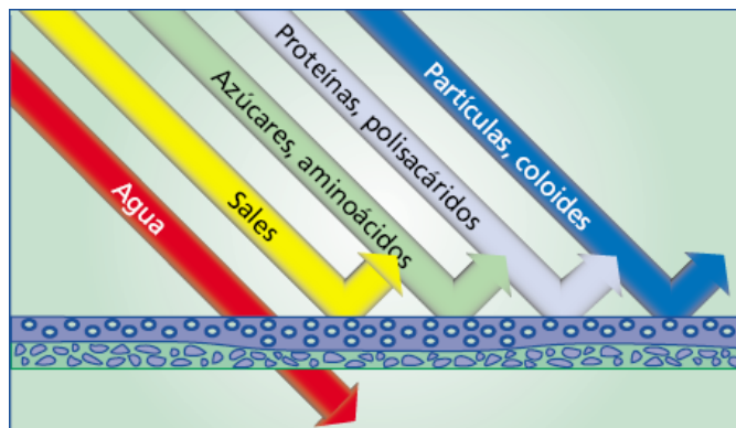
Figura 8. Componentes retenidos por la membrana en la OI. Fuente: GEA (2007).
