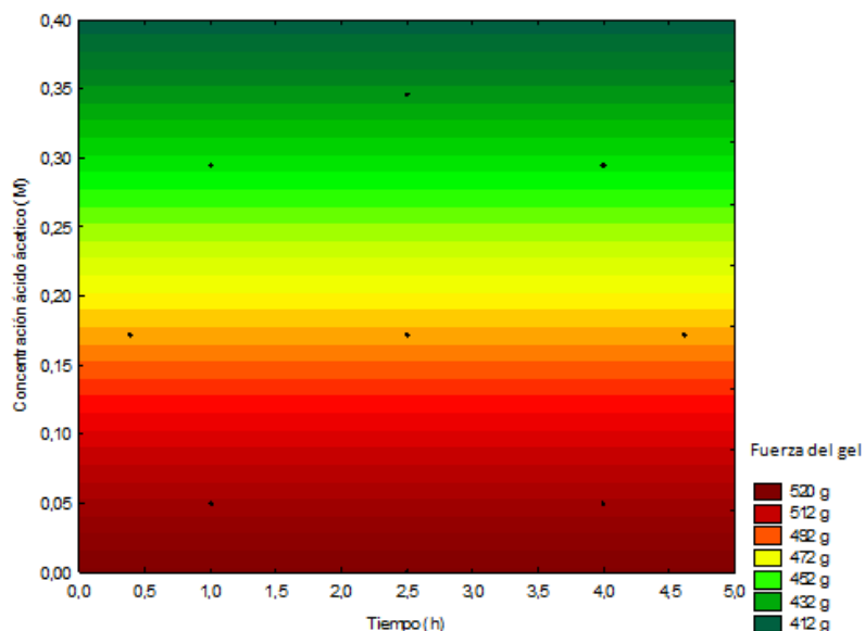
Figura 23. Efecto de la concentración del ácido acético sobre la fuerza del gel elaborado con la proteína extraída de la piel de atún.
