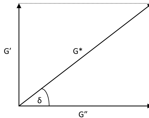
Figura 7. Diagrama vectorial de la relación entre G' , G'' y G^* .
