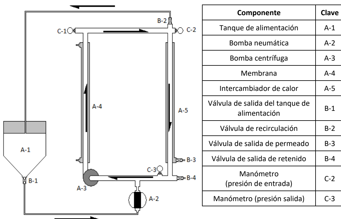
Figura 19. Diagrama del equipo de MFT/UFT.
